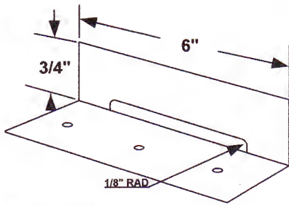
18 GA GALV. SLIDER CLIP BASE
